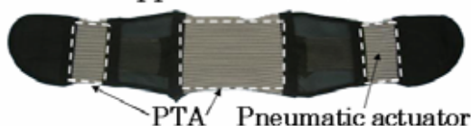
図1 アクティブサポータの構造(プロトタイプ)
